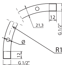
尺寸图
