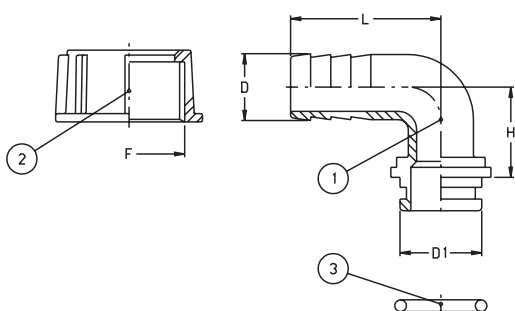
90度弯管快接头
